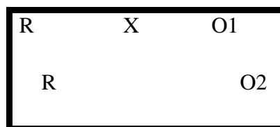
Gambar 3.1. Desain Penelitian
